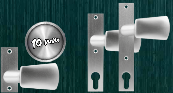
ARTIKEL 45480 Schraubenabstand: 67 mm / 67 mm / 105 mm
