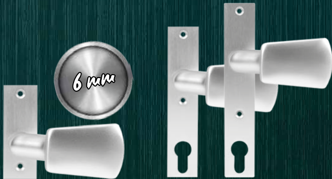
ARTIKEL 45410 Schraubenabstand: 67 mm / 67 mm / 105 mm
