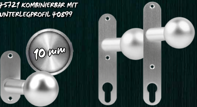
ARTIKEL 45721 Schraubenabstand: 67 mm / 67 mm / 105 mm
