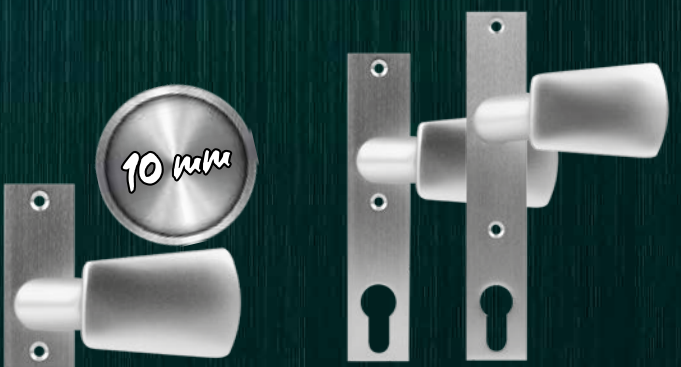
ARTIKEL 45718 Schraubenabstand: 67 mm / 67 mm / 105 mm
